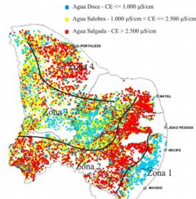
Figura 1. Qualidade da água subterrânea no domínio das rochas cristalinas dos estados do CE, RN, PB e PE. Valores de condutividade elétrica medidos in loco em poços tubulares.
