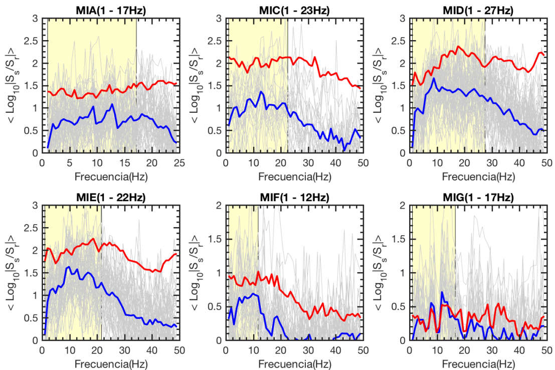
Figura 3.4.- Aplicación de la SSNR a todos los datos y por estación. La parte sombreada en amarillo, corresponde a la banda espectral seleccionada por estación.
