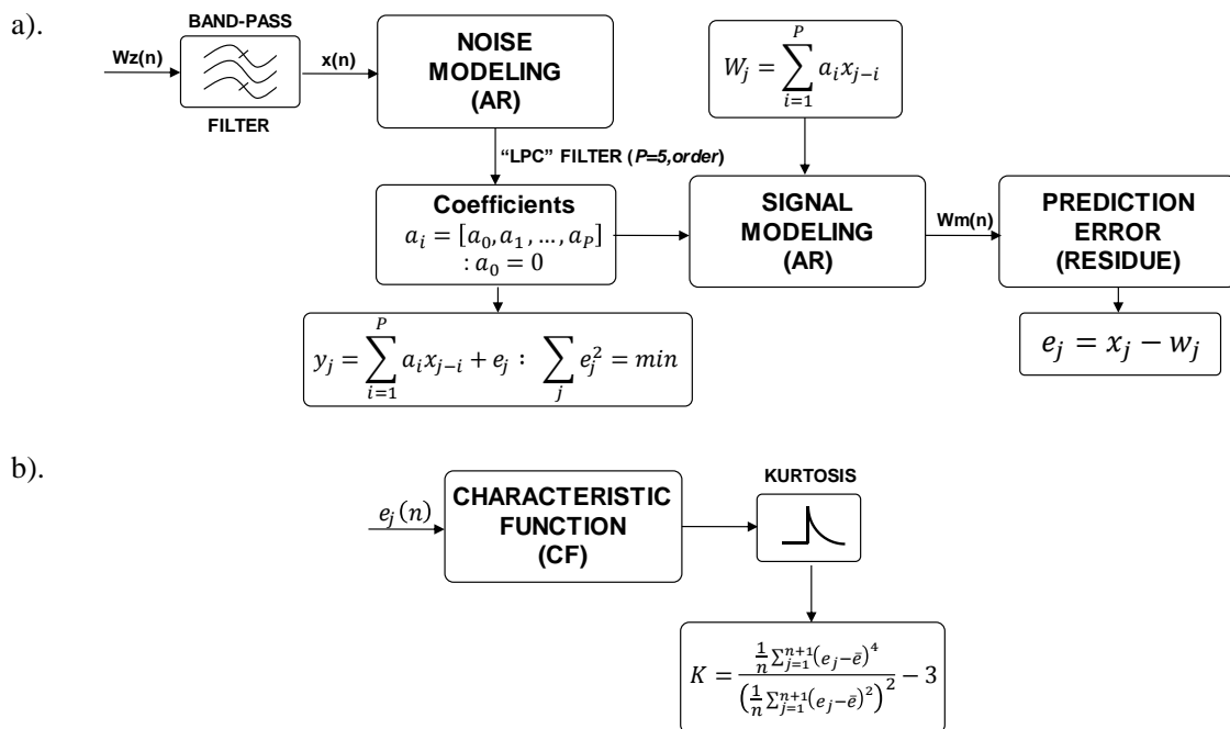
Figura 3.12.- Diagrama de bloques que ilustra (a) la estimación del error de predicción de un proceso autorregresivo (AR) y b) la segunda parte del proceso que corresponde al cálculo de la CF, utilizando la curtosis.
