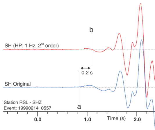
Figura 2.6.- Efecto de un filtro paso-alto Butterworth de 2º orden (1 Hz) en un registro de período corto. En este ejemplo, el filtro provoca un cambio significativo en la forma de onda (Diehl et al., 2012).
